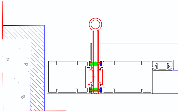
DOBRADIÇA DE BALANÇO TRIPLA DOB-BR01T
