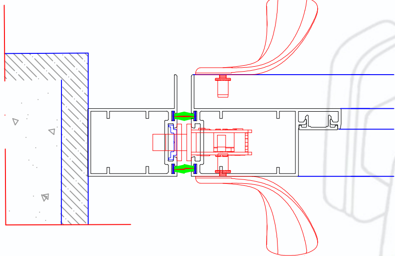
FECHADURA BICO DE PAPAGAIO PUXADOR ESQ / DIREITO CILINDRO EUROPEU
