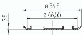
CORTE B-B
