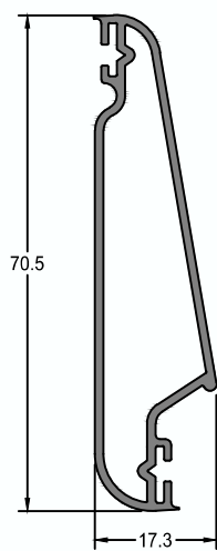
Pefil PT-01
