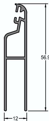
Pefil PT-02
