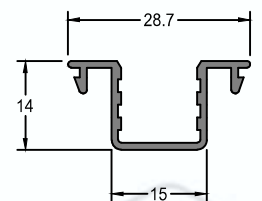
Pefil PT-03
